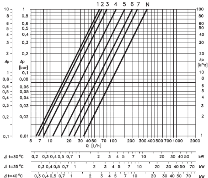
Diagram för ventilinsats Danfoss RA-U, Gul Kv-värde, RA-U 013G0373: 0,04-0,24
