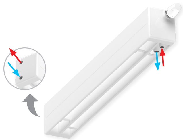
Serieanslutning med tillopp/retur höger botten SEH
