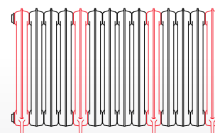
720 x 1180 14 sektioner (4+10)
