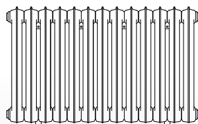
660 x 1098 13 sektioner
