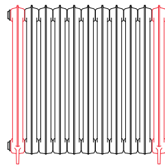
920 x 934 11 sektioner (3+8)
