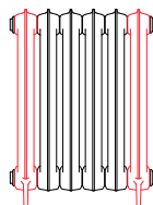
720 x 524 6 sektioner (2+4)
