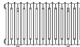
560 x 1016 12 sektioner
