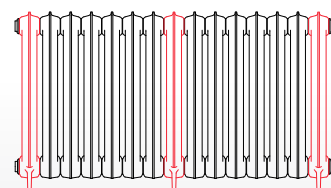
720 x 1262 15 sektioner (3+12)
