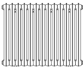
860 x 1098 13 sektioner
