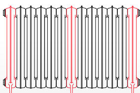
720 x 1098 13 sektioner (3+10)
