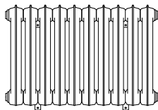
560 x 852 10 sektioner
