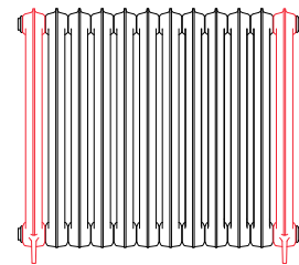
920 x 1016 12 sektioner (4+8)
