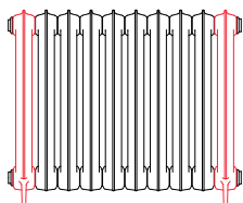
720 x 852 10 sektioner (2+8)
