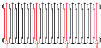
620 x 1344 16 sektioner (4+12)
