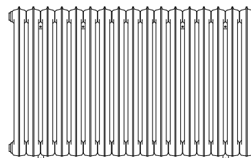
860 x 1426 17 sektioner
