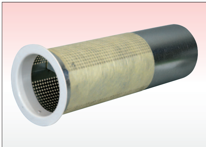
Kanal i perforerad plåt med eller utan ljudbaffel. Finns i dimensionen Ø100 mm med eller utan ljudbaffel. Längd 350 mm, Andra längder kan fås vid begäran.
