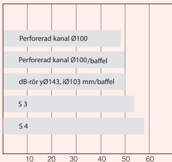
Ljuddämpning Dn, e, w (dB)
