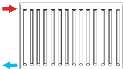
Modul Compact Hygien – sidoanslutning.
